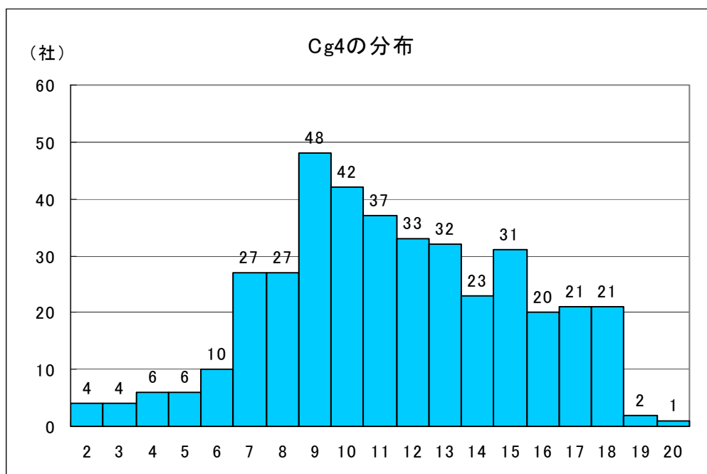
Cg4 の分布
