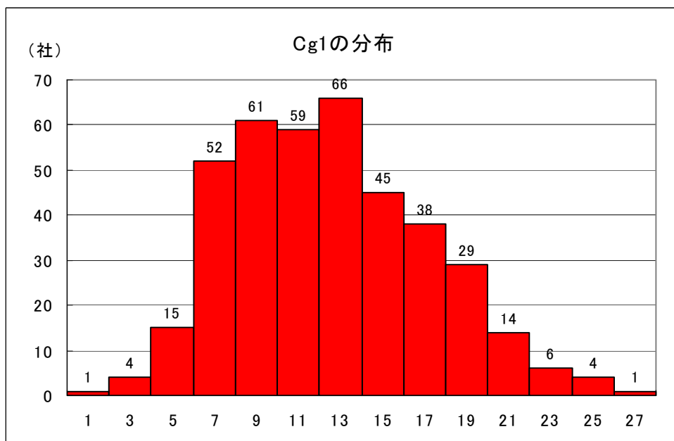
Cg1 の分布
